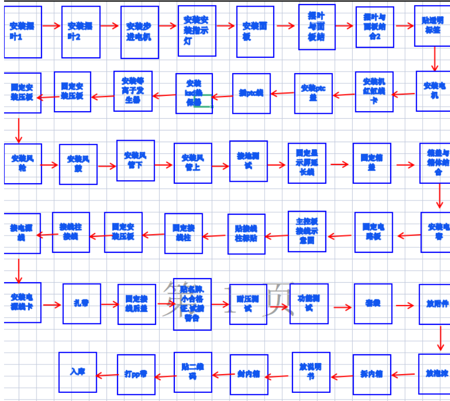
图 3-2 工艺流程图
